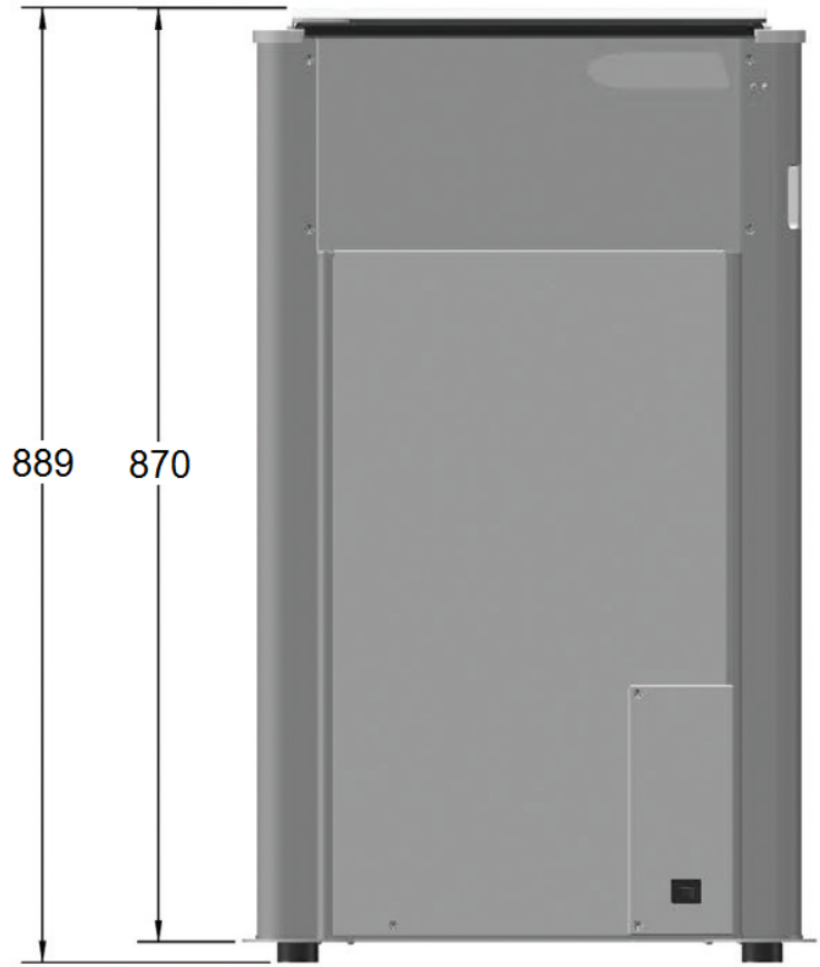
Frontansicht
