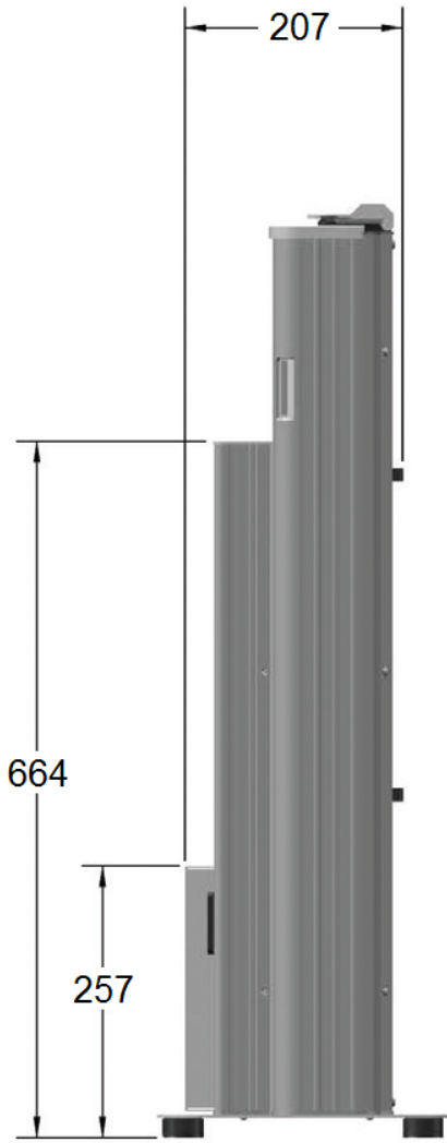
Seitenansicht
